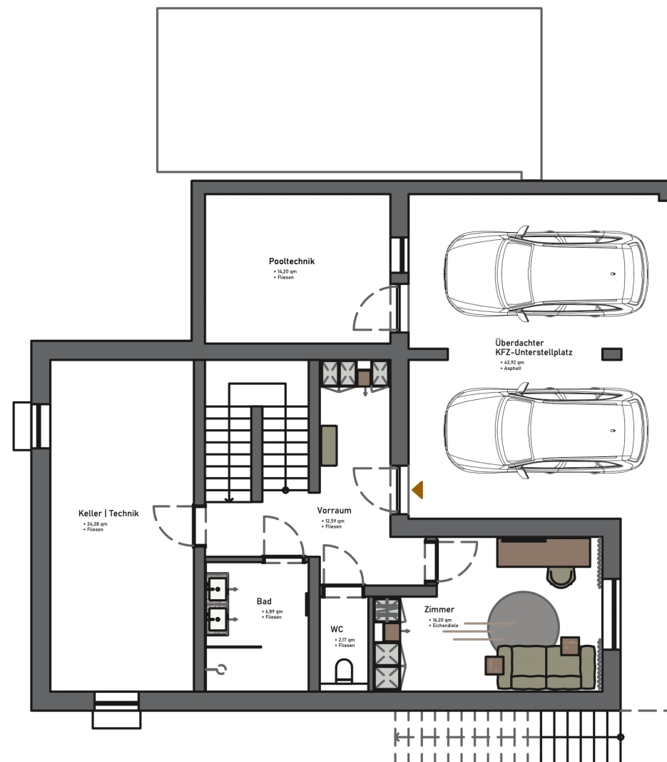
Kellergeschoss M 1 : 200
